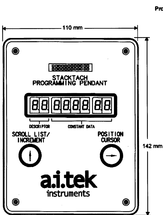
Programming Pendant
